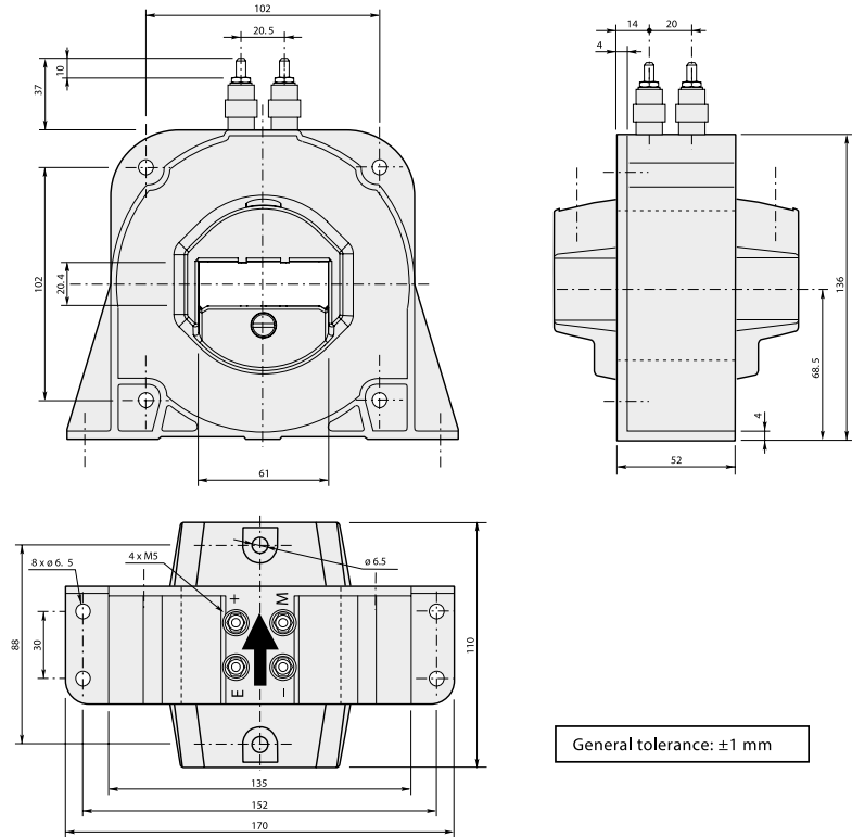
Size 2 - CS2000BRV and HRS2000-T-014 / HRS2500-T-014
